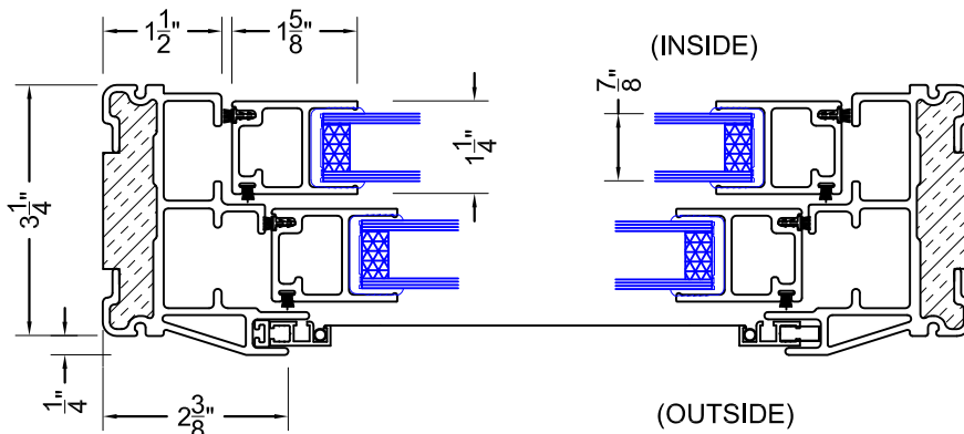
JAMB DETAIL
