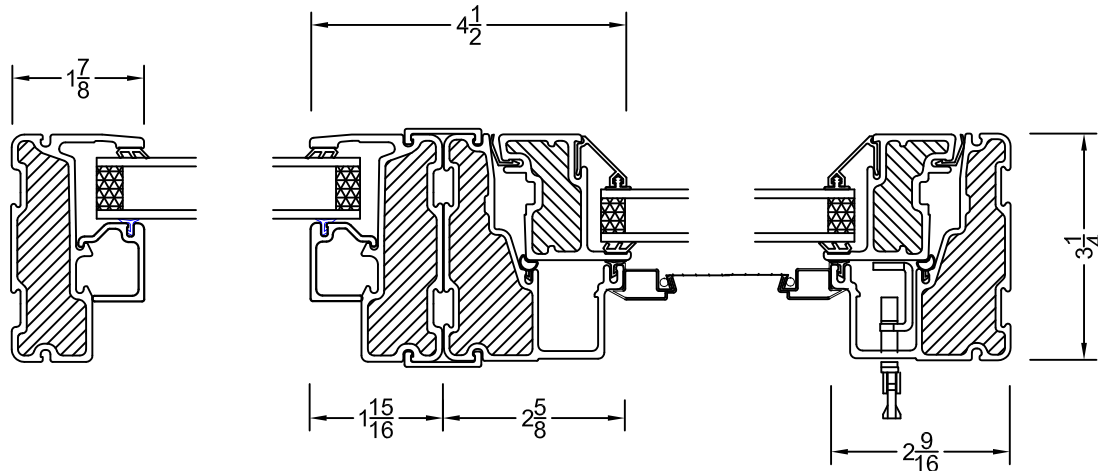
JAMB DETAIL
